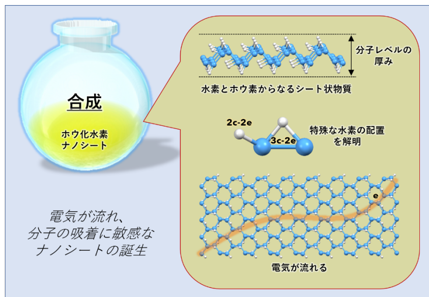
図：ホウ化水素ナノシートを化学的に合成。分子レベルの厚みのシート状物質で、特殊な水素の配置を有する。電気が流れ、その導電性は分子の吸着に敏感。
