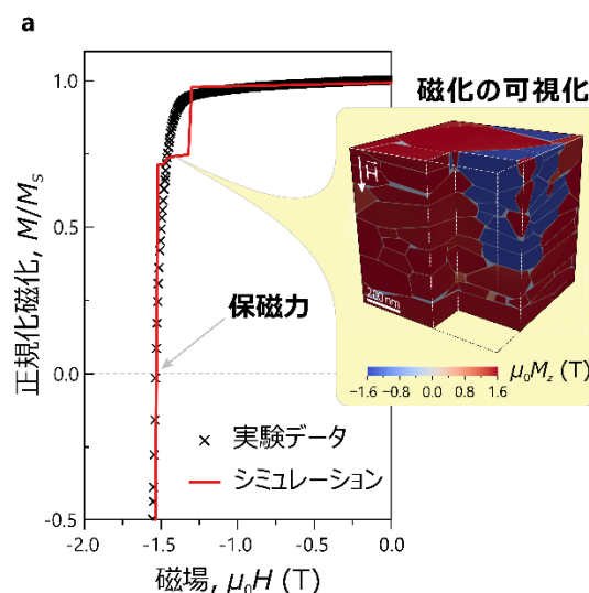
図 2 トモグラフィーに基づくモデルを用いたマイクロマグネティックシミュレーション。(a)FIB-SEM トモグラフィーを行った熱間加工ネオジム磁石の第 2 象限における減磁曲線のシミュレーションと実験データ。減磁曲線上の 1 点における磁区分布を挿入図で示す。
